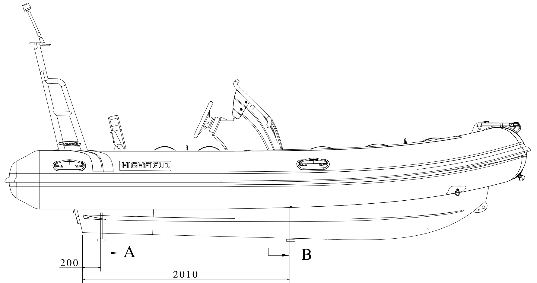
LONGITUDINAL PROFILE
